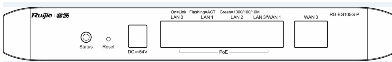
图 1-2 RG-EG105G-P 出口网关产品后面板
