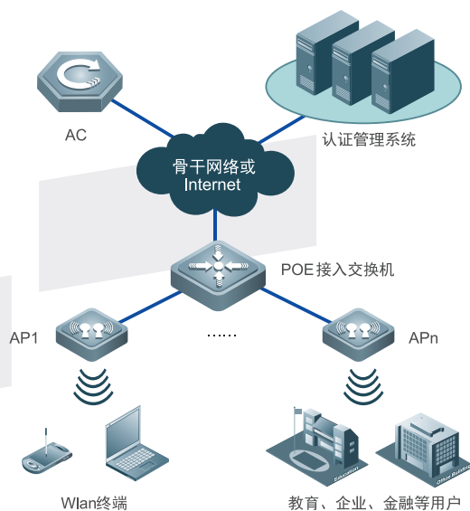
RG-RAP220(EV2)典型组网示意图：
